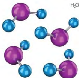
Shluky molekul vody
